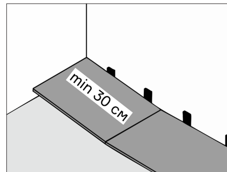
Рис. 5 Укладка последней плитки ряда
