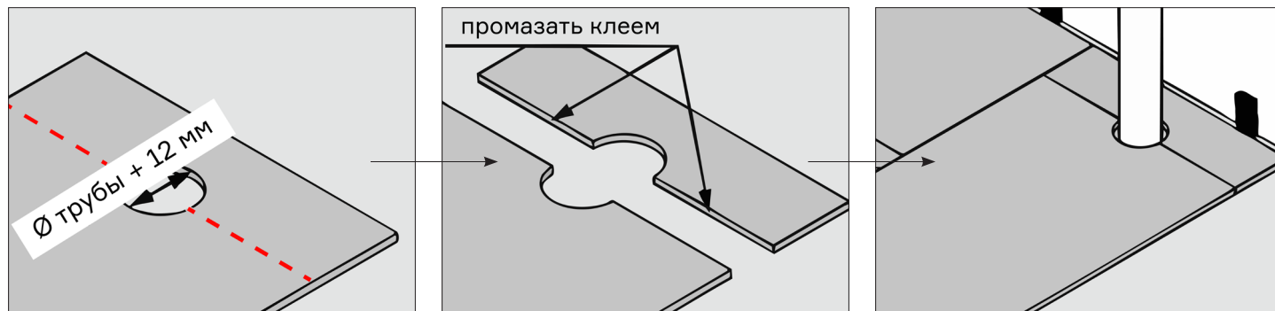
Рис. 10 Обход трубы
