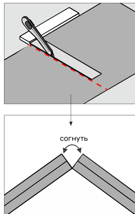
Рис.2 Подрезка плитки при помощи строительного ножа
