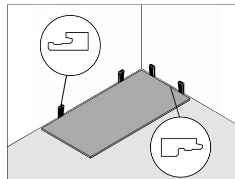
Рис. 3 Укладка первой плитки
