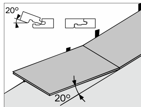
Рис. 4 Укладка следующих плиток первого ряда
