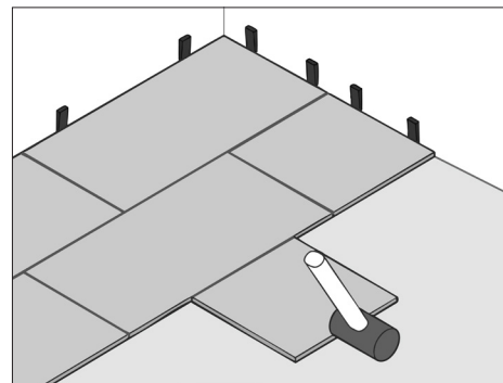
Рис. 7 Подбивка плиток второго ряда
